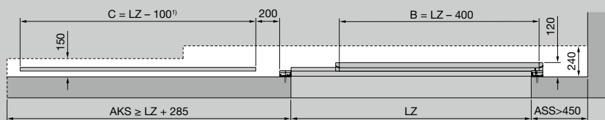
Montaje en el techo B (sección de la guía del suelo)
