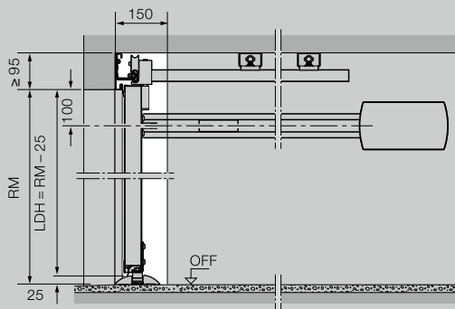
Automatismo montado en la pared
