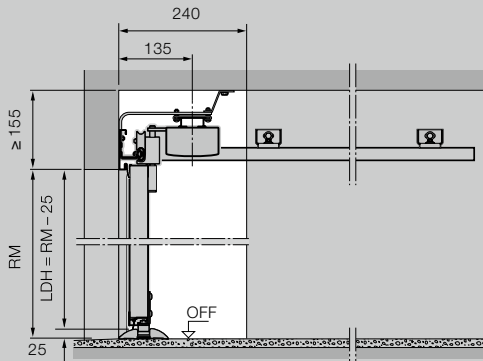
Automatismo montado en el techo
