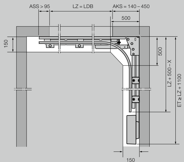
Guías ES (carril sencillo, automatismo montado en el techo A)
